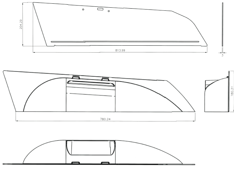
Fig. 14. Sketch costruttivi di fiancate interne removibili e scambiabili di una stessa sega squadratrice: fiancata piana (alto) e bombata (basso) aventi spessore minimo di 3 mm
