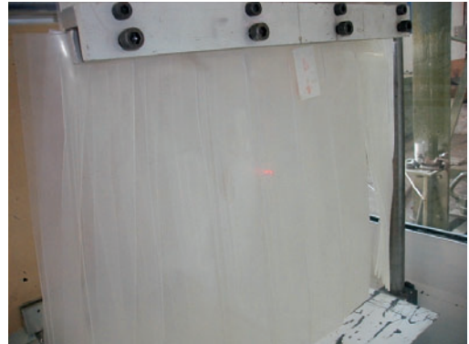
Fig. 4b. Sistema di puntamento laser per centrare la canna nel punto desiderato del provino (questa immagine di repertorio mostra una protezione realizzata con cortine flessibili sottoposta a prova).
