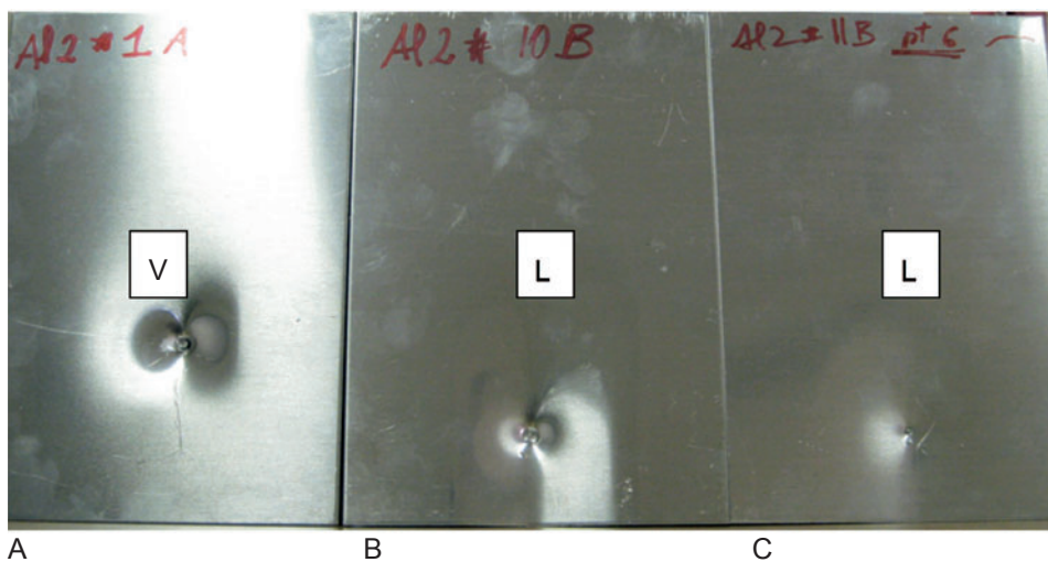
Fig. 25. Confronto fra provini da 2 mm dopo l'impatto con punta tronco-conica nel punti V (A) e L (B) e con punta conica in L (C)
