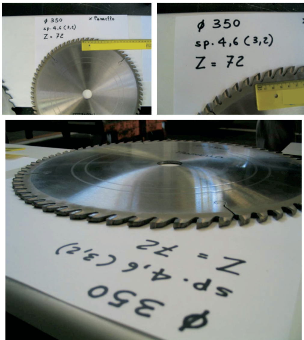
Fig. A1.5. Sega per pannello - diametro 350 mm
