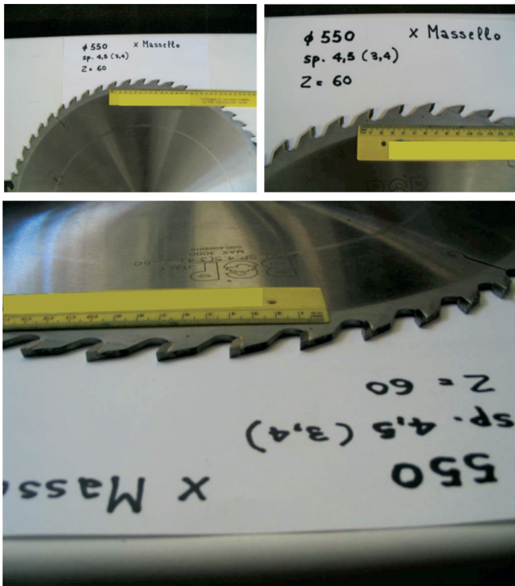
Fig. A1.2. Sega per massello - diametro 550 mm
