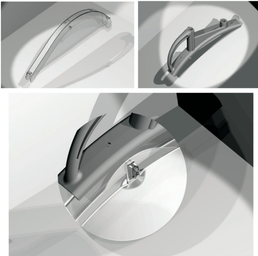
Fig. 12. Dettagli della protezione di Fig. 11: cuffia (in alto-sinistra), maniglia (in alto-destra) ed particolare dell'aggancio cuffia-maniglia.
