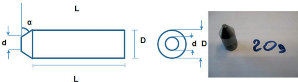
Fig. 9. Proiettile cilindrico calibro 12 mm a punta tronco-conica costruito in acciaio e con massa di 20 g
