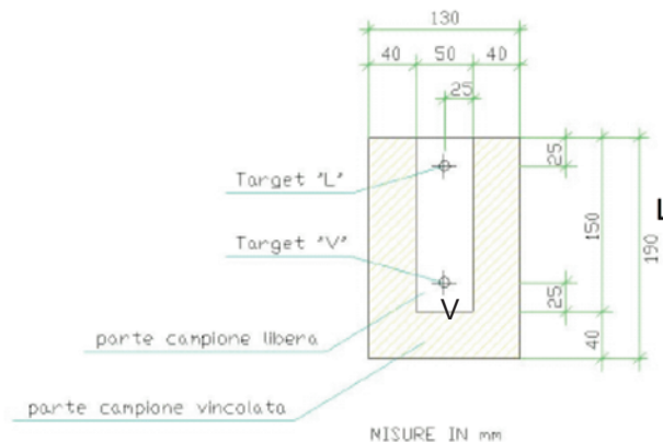
Fig. 15. Sketch quotato della configurazione di prova alternativa a quella della norma, al fine di realizzare test di impatto più localizzati; la mascherina ad "u" determina sul provino una striscia di prova nella mezzeria della quale sono indicati con L e V i due punti di impatto prescelti.
