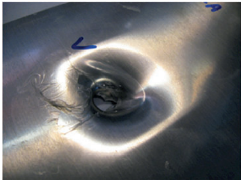
Fig. 21. Prova A4 con bozzatura perforante dell'alluminio usando un proiettile conico da 20 g.
