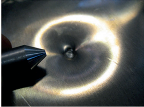
Fig. 20. Prova A3 con bozzatura NON perforante dell'alluminio usando un proiettile conico da 20 g.
