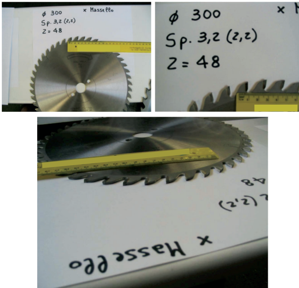
Fig. A1.1. Sega per massello - diametro 300 mm
