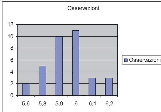
Fig. 24. Istogramma delle misure di velocità in Tab.6. Il diagramma prova e quantifica l'effetto delle dissipazioni in termini di riduzioni di velocità del proiettile all'impatto. La media delle registrazioni è infatti di 5.9 m/s, un dato inferiore di circa il 2,5% rispetto al valore teorico richiesto a meno delle frizioni e dissipazioni pari a V_{teorica} = 6.26 m/s
