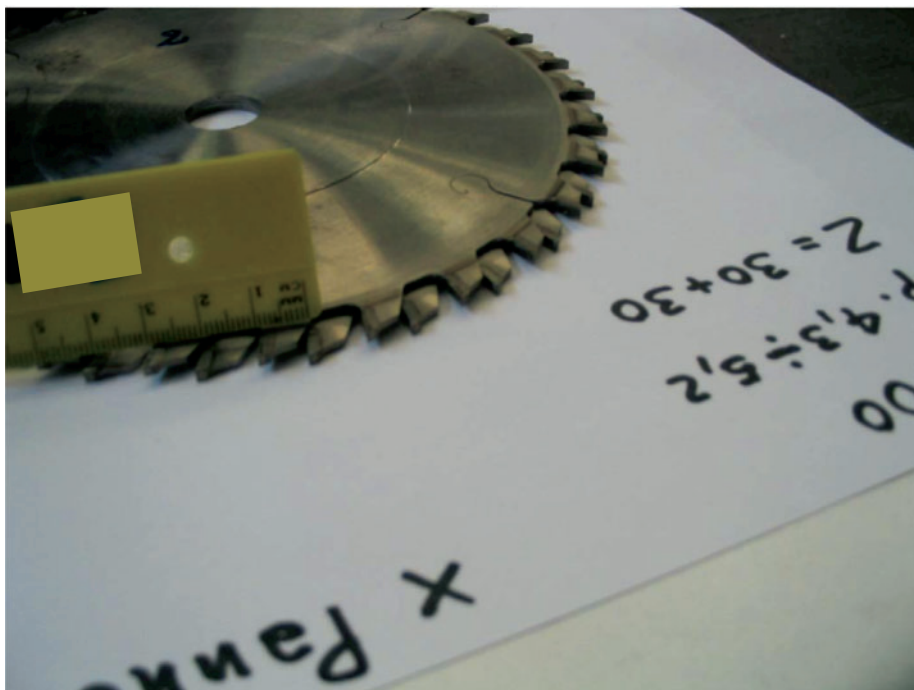
Fig. A1.4. Sega per pannello - diametro 200 mm
