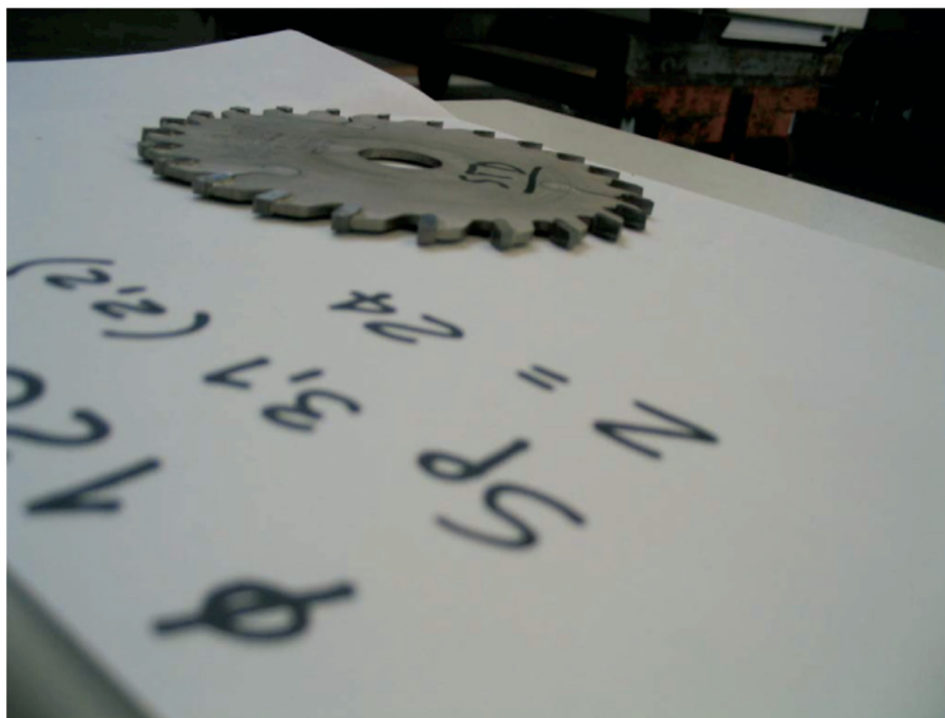
Fig. A1.3. Sega per pannello - diametro 120 mm
