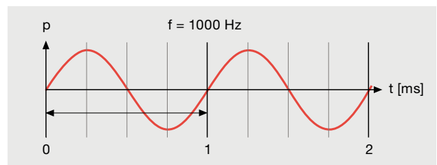
5 Periodo e frequenza: oscillazione di periodo T = 1 \text{ ms} = 1000 oscillazioni al secondo = 1000 Hz.
