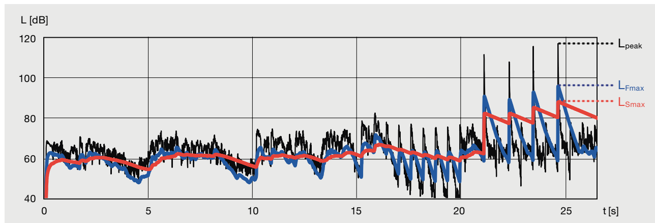
47 Valore massimo «peak» e valori effettivi «fast» e «slow» di un segnale acustico.
